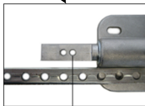
Riegelstange kürzen
